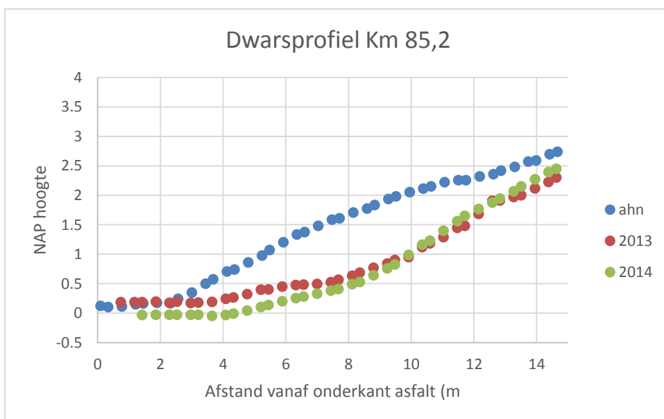
Figuur 14 – Vergelijking hoogteprofielen van 2014, 2013 en AHN-2 bij km 85,2
