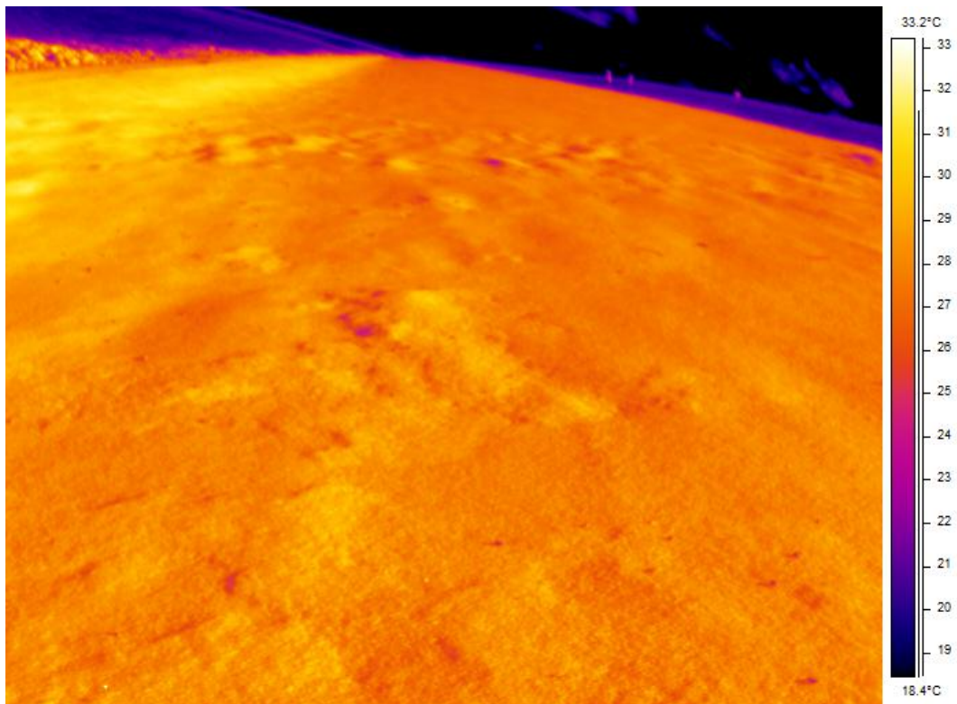
Figuur 9 – Warmtebeeld met opbollingen bij km 85,1
