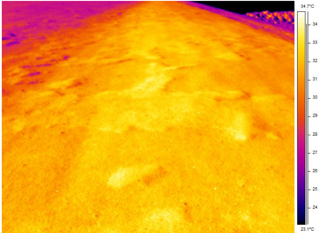
Figuur 10 – Warmtebeeld met opbollingen bij km 85,0
