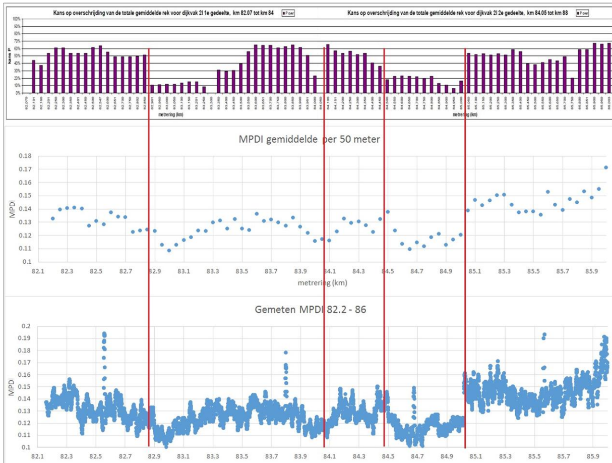
Figuur 13 – Vergelijking methoden voor sterktebepaling d.m.v. VGD en MIRA
