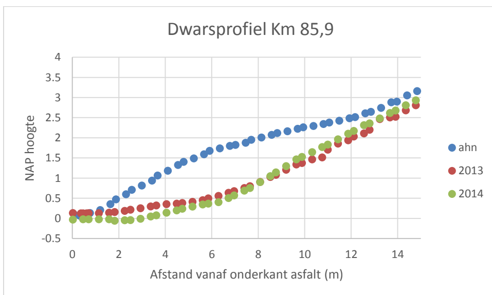
Figuur 15 – Vergelijking hoogteprofielen van 2014, 2013 en AHN-2 bij km 85,9
